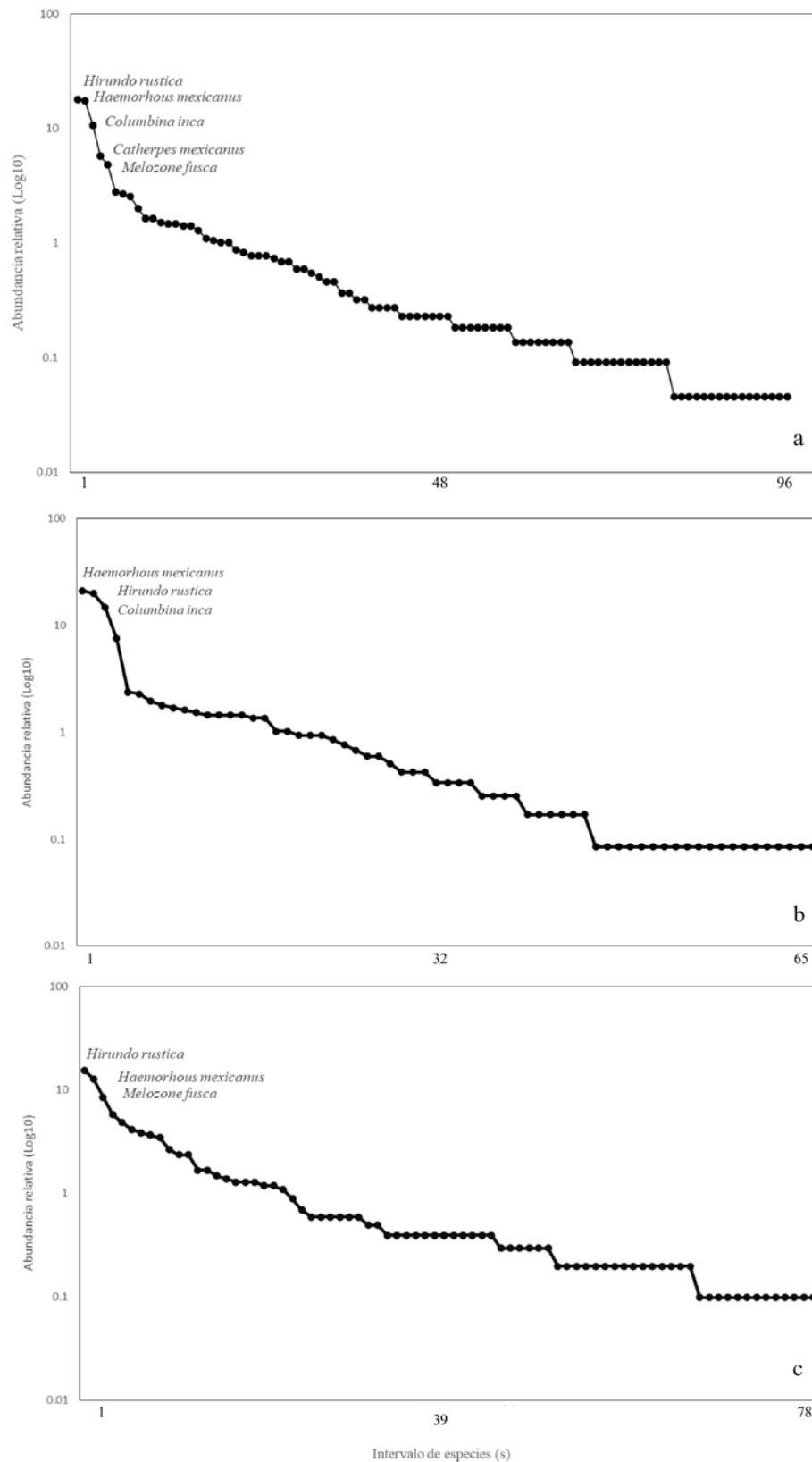
Figura 4. Curva rango-abundancia de las especies de aves de la Sierra de Santa Catarina, Ciudad de México Marzo del 2022 a febrero del 2023. a = Curva rango-abundancia de las especies de aves presentes en ambos tipos de vegetación, b = Curva rango-abundancia de las especies de aves presentes en el matorral, c = Curva rango-abundancia de las especies de aves presentes en el pastizal.
