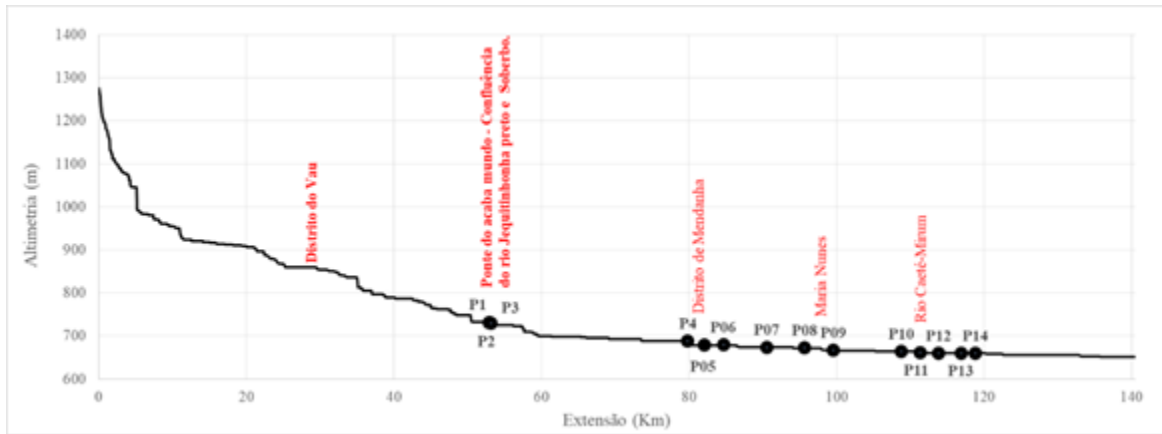
Figura 7: perfil longitudinal do Rio Jequitinhonha, apresentado as localidades e os pontos de controle Fonte: Autores, 2019.
