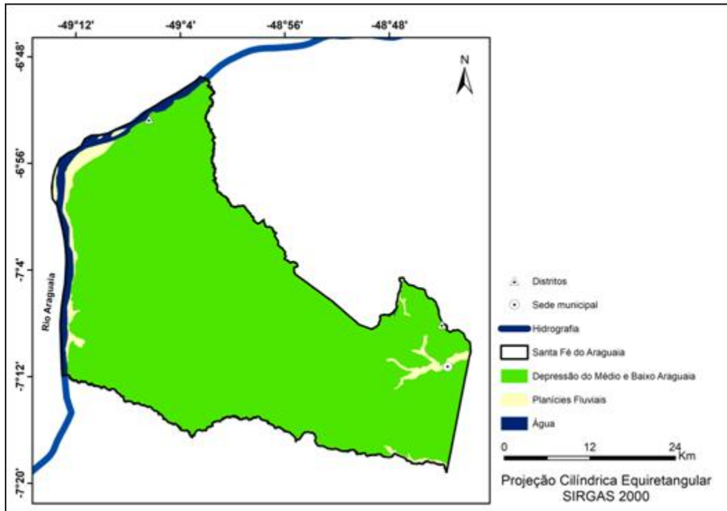
Figura 2 – Geomorfologia do município de Santa Fé do Araguaia Fonte: Autores (2021).
