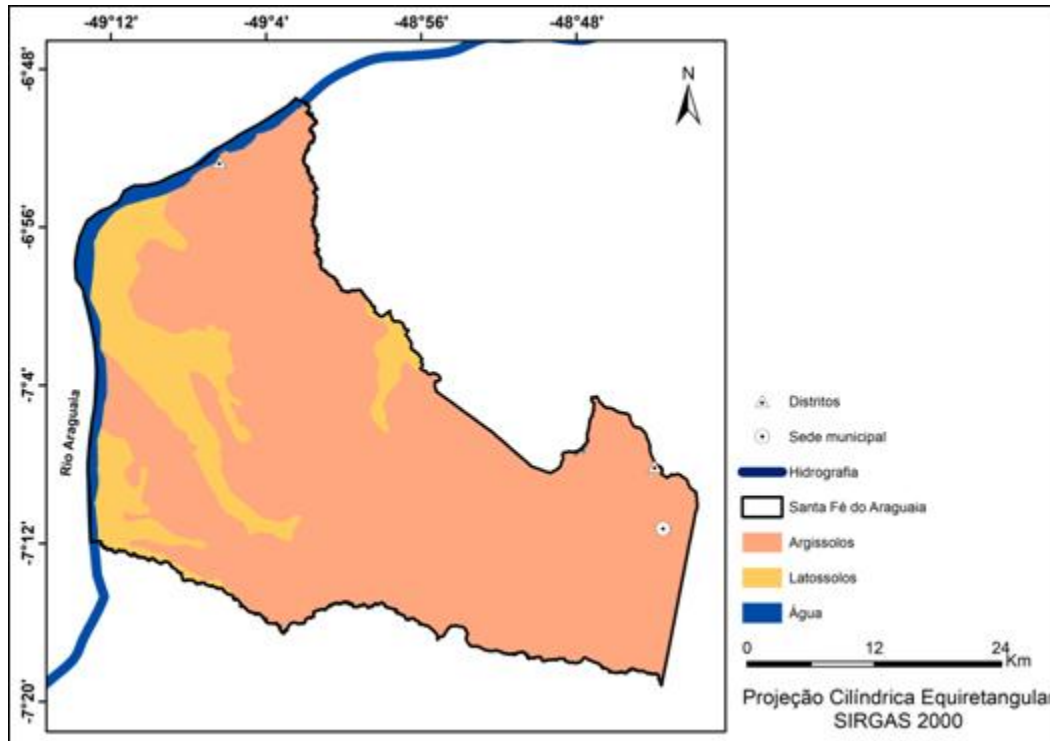
Figura 4 – Classes de solo no município de Santa Fé do Araguaia Fonte: Autores (2021).
