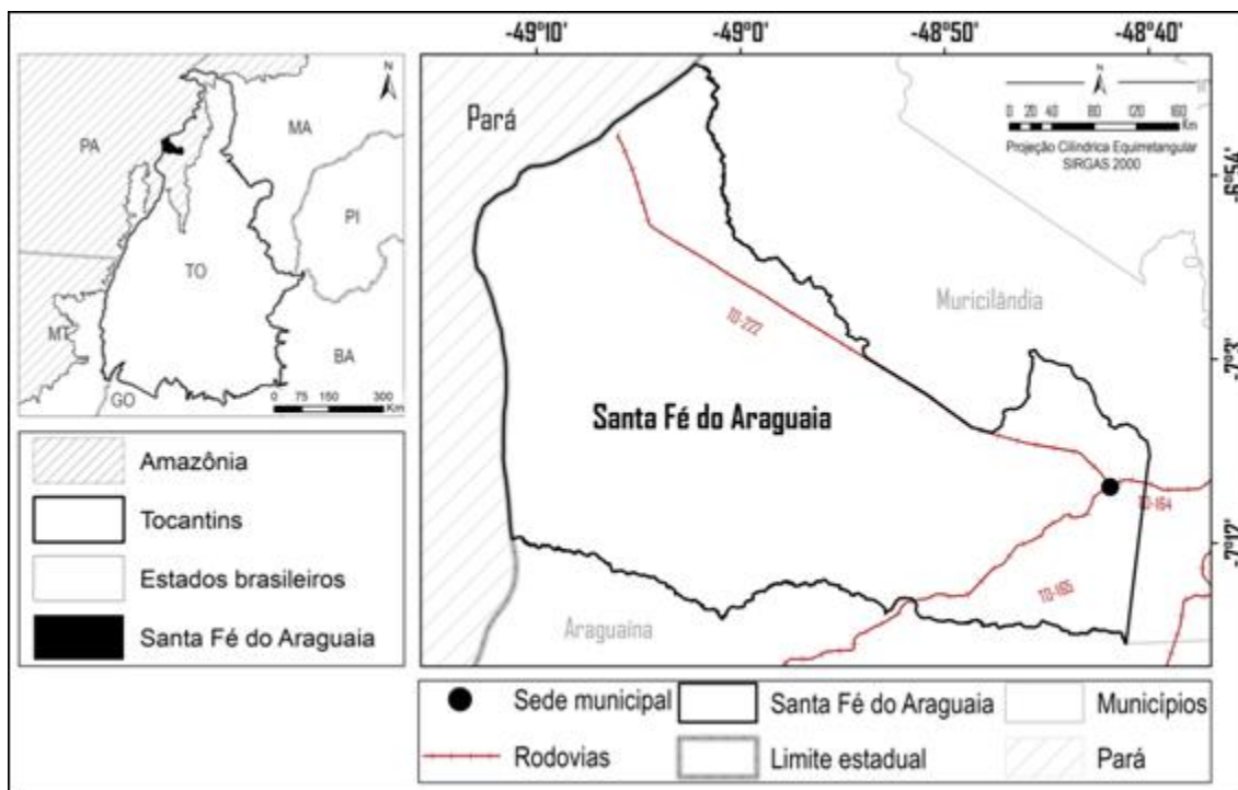
Figura 1– Localização do município de Santa Fé do Araguaia/Tocantins Fonte: Webber (2024).
