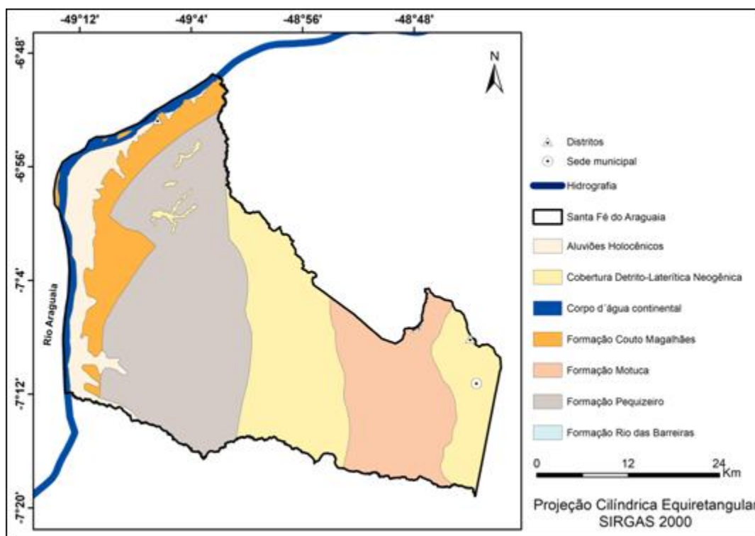
Figura 3 – Geologia do município de Santa Fé do Araguaia Fonte: Autores (2021).
