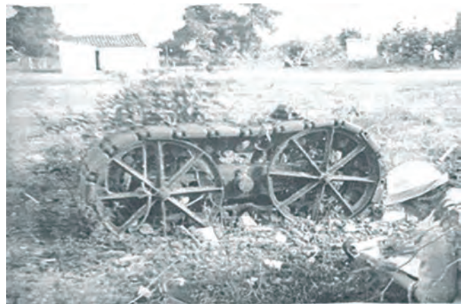
FIGURA 8. Sistema de rodaje de una carreta CATERPILLAR (Rodríguez, 1999).
