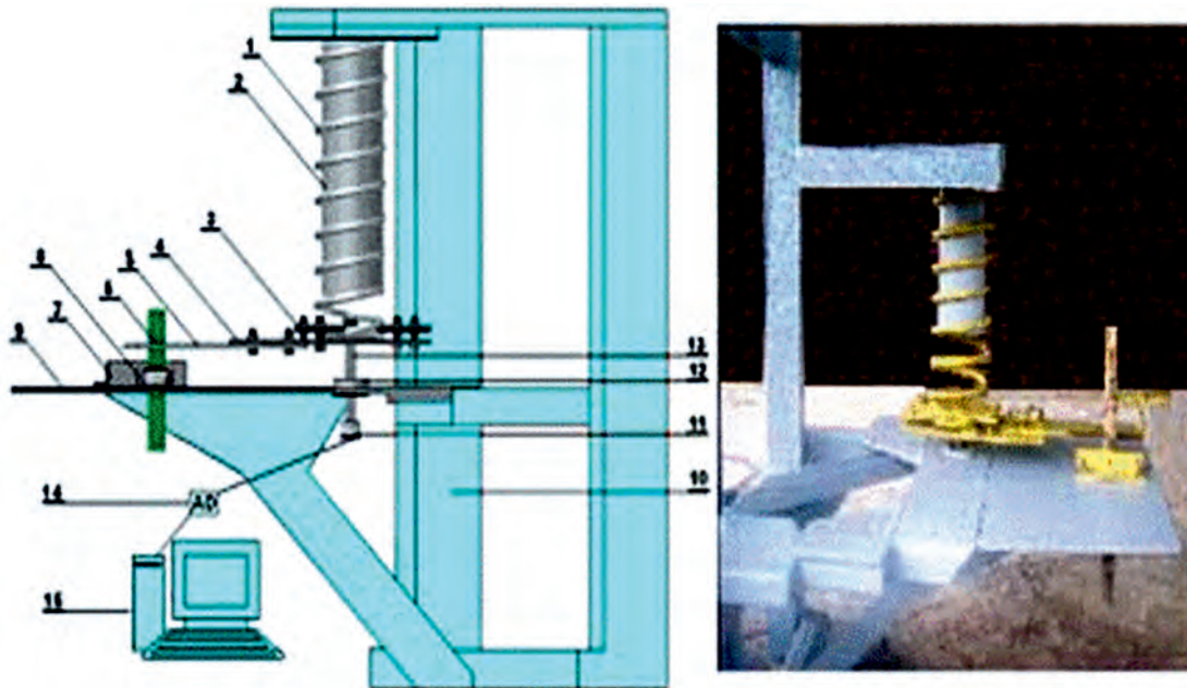
FIGURA 2. Instalación empleada durante la medición de la energía específica de corte, fuente: Valdés e Iglesias (2002a) y Valdés et al. (2008)
