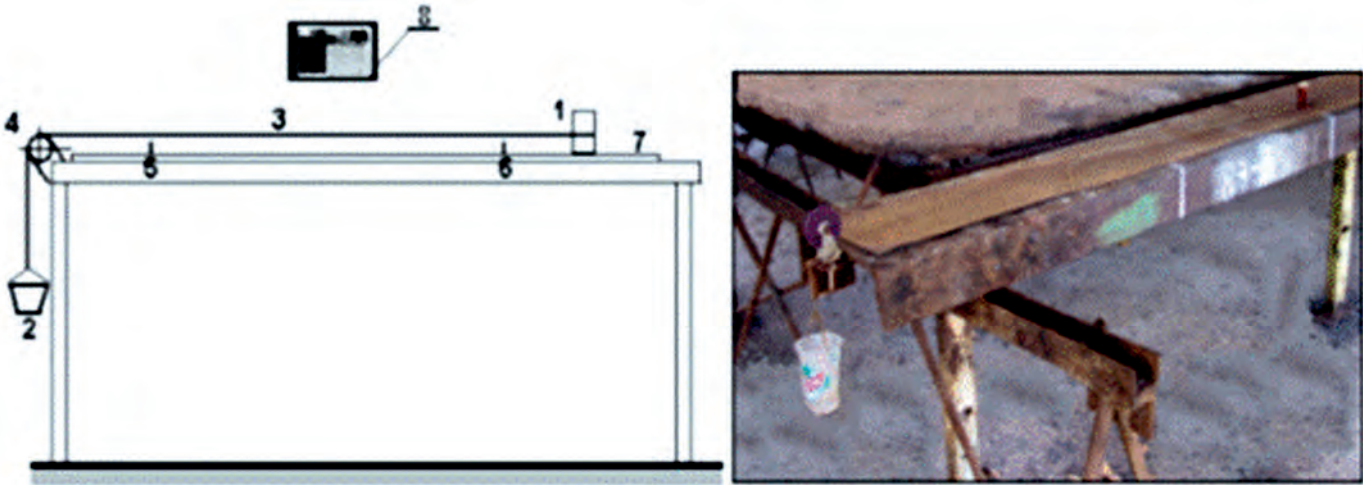
FIGURA 1. Instalación mecánica que se emplea en los ensayos, fuente: Valdés e Iglesias (2002a) y Valdés et al. (2008). Leyenda: 1 - Muestra. 2 - Peso conocido. 3 - Hilo. 4 - Polea. 5 y 6 - Marcas de cronometraje. 7 - Plancha de acero. 8 - Cámara de video.
