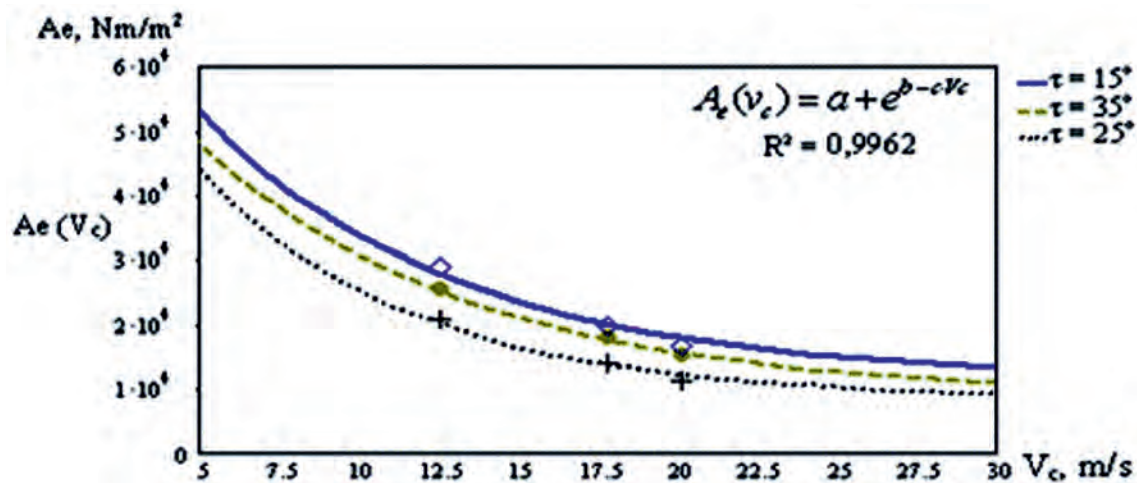
FIGURA 3. Variación de la energía específica durante el corte de los tallos en función de la velocidad de corte, para los diferentes ángulos de deslizamiento, ajustadas al modelo exponencial, fuente: Valdés (2008).
