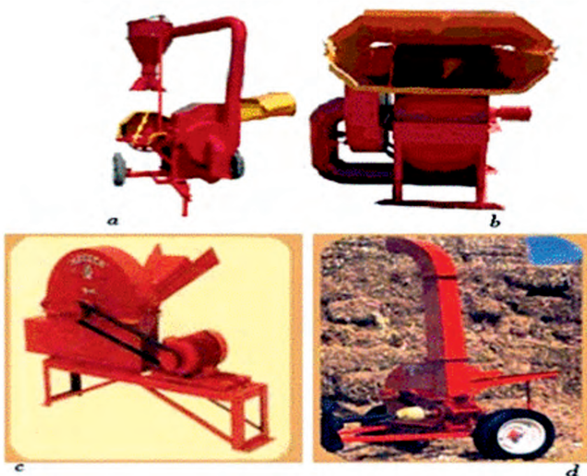
FIGURA 6a). Modelo 18-32, b) Modelo 20-36, c). Picadora de forraje eléctrica modelo AZTECA, d). Picadora de forraje para acoplar a tractor modelo AZTECA, fuente Valdés (2008).
