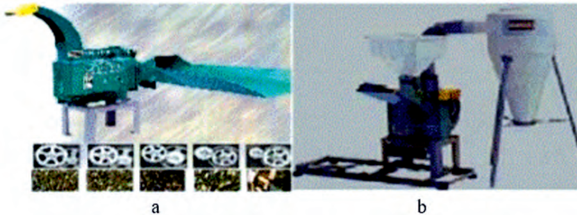
FIGURA 5a). Modelo EN-12, b). Modelo DPM-4, fuente: Valdés (2008).
