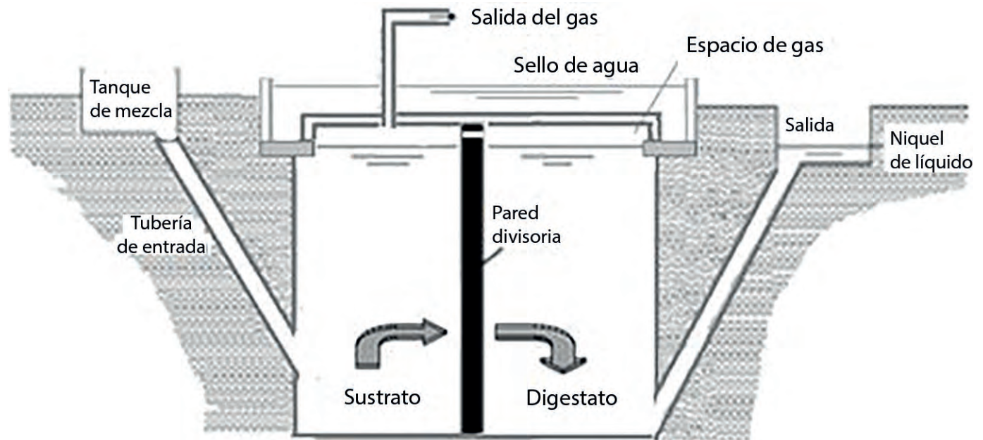
FIGURA 4. Esquema general de un biodigestor híbrido cubano (Hermida, 2014).
