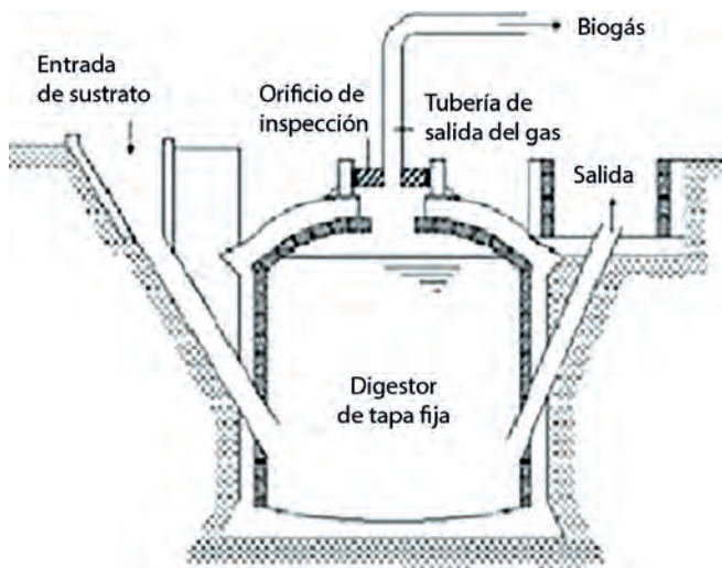
FIGURA 1. Esquema general de un biodigestor de tapa fija o de tipo Chino (Santerre & Smith, 1982)
