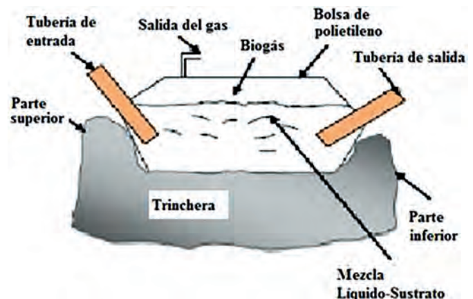
FIGURA 3. Esquema general de un biodigestor tubular o de bolsa de polietileno (Frederiks, 2011).
