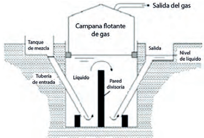
FIGURA 2. Esquema general de un biodigestor de campana flotante o de tipo Hindú (Group, 2007)
