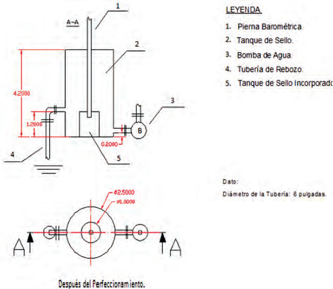
FIGURA 2. Tanque de sello del filtro rotatorio al vacío después del perfeccionamiento.
