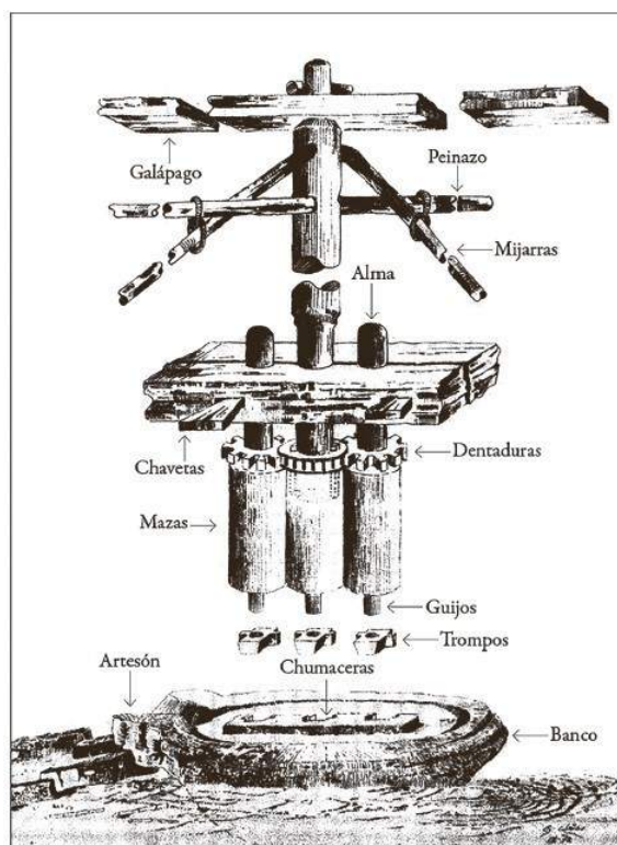
Figura 10 – Elementos de un trapiche de madera
