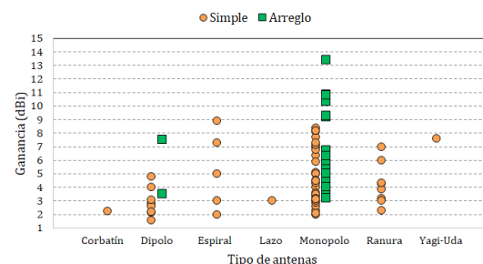
Figura 5. Ganancia máxima de las antenas.
