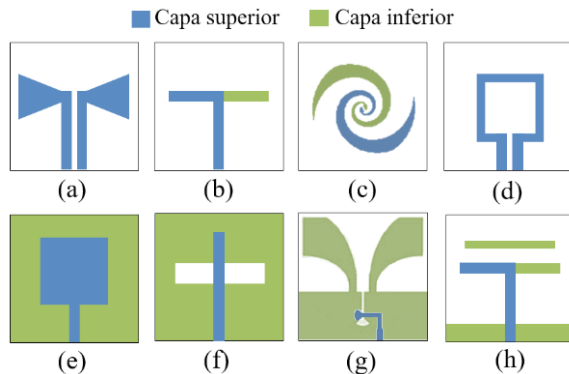
Figura 3. Configuración básica de las antenas empleadas: a) corbatín, b) dipolo, c) espiral, d) lazo, e) monopolo, f) ranura, g) vivaldi y h) yagi-uga.
