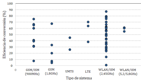
Figura 2. Eficiencia de conversión máxima en función de los sistemas RF.
