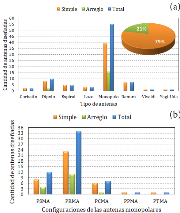
Figura 4. a) Antenas usadas en las rectenas y b) formas de parche de las antenas monopulares.
