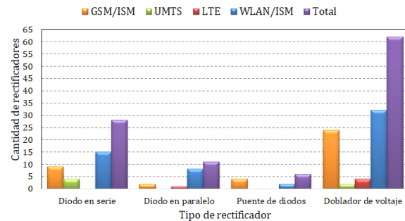
Figura 6. Tipos de rectificadores utilizados en las rectenas por sistema de comunicación.
