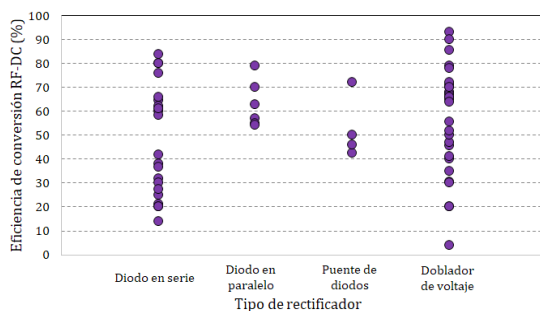
Figura 7. Eficiencia de conversión RF-DC máxima por cada tipo de rectificador.
