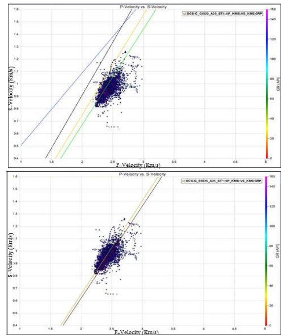
Figura 2. Gráfico de correlación cruzada de velocidad P versus velocidad S en el Pozo OCS-G_05825_A25_ST1. Código de colores: Registro de rayos gamma.
