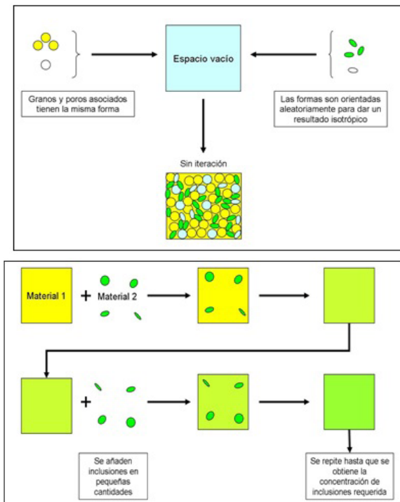
Figura 3. Ilustración del método Autoconsistente y de Xu y White (basado en el modelo de Medio diferencial efectivo).
