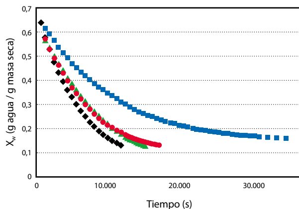
Figura 3. Curvas de secado experimentales para las distintas condiciones de Temperatura ( T ) y humedad relativa (HR) del aire de secado. (▲) T=30 °C, HR=40%; (■) T=30 °C, HR=80%; (◆) T=50 °C, HR=40%; (●) T=50 °C, HR=80%.
