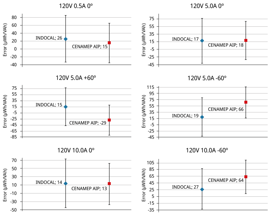
FIGURA 2. Resultados generados por los dos laboratorios participantes (donde 0° representa un factor de potencia unitario; +60° es un factor de potencia 0.5 capacitivo; y, -60° es un factor de potencia 0.5 inductivo).
