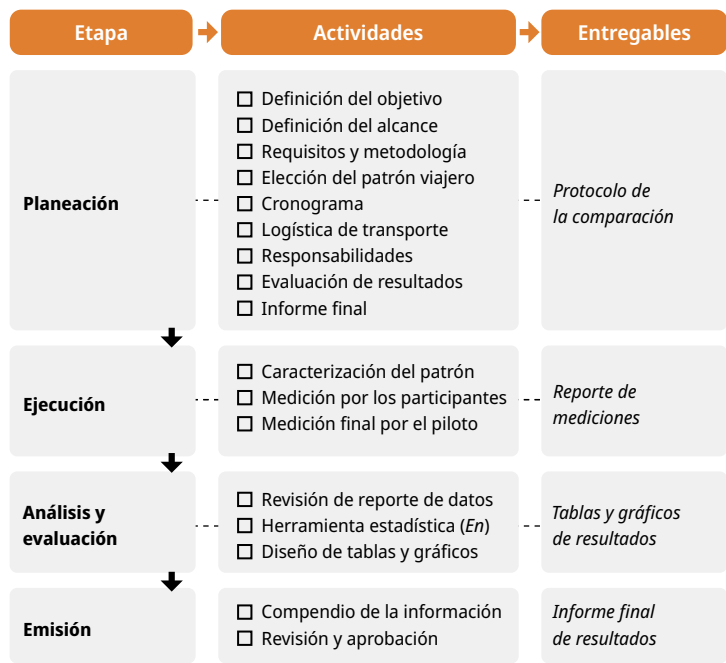
FIGURA 1. Esquema simplificado del proceso realizado en la comparación interlaboratorio en los dos países.
