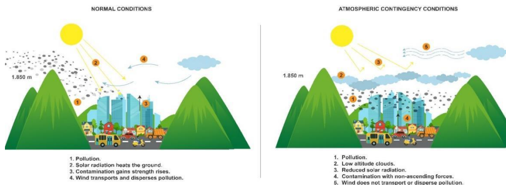
Figura 3. Condiciones normales y de contingencia atmosférica resultante de las condiciones meteorológicas en el Valle de Aburrá. Valle de Aburrá, Colombia.
