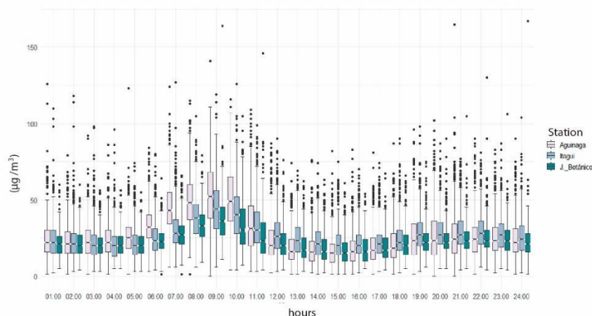
Figura 4. Promedio horario PM 2.5 ( \mu\text{g}/\text{m}^3 ). Estaciones de calidad del aire. Valle de Aburrá, Colombia. 2009 – 2011
