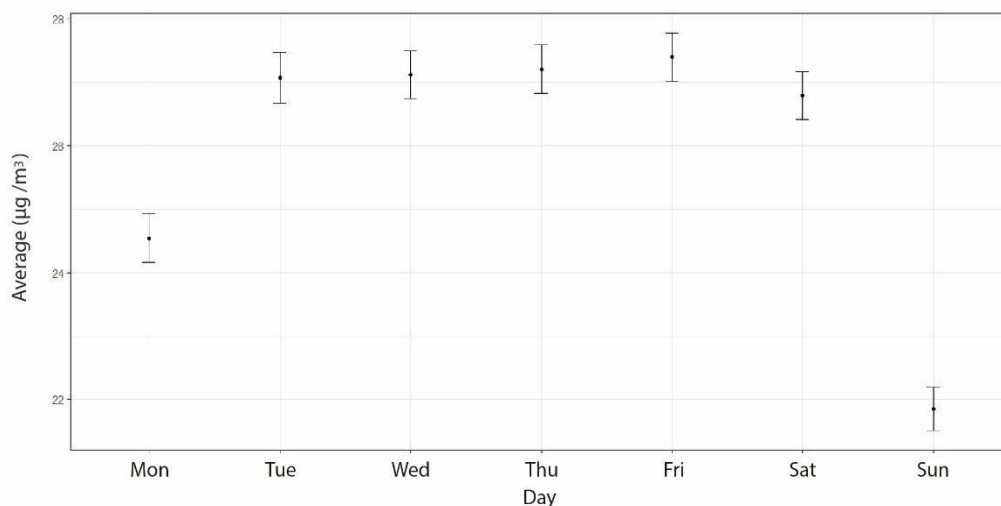
Figura 7. Intervalos de confianza PM 2.5 promedio (µg /m 3 ) por día de la semana Valle de Aburrá, Colombia. 2009 - 2011.
