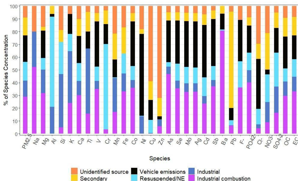
Figura 10. Huellas de perfil de fuentes en la estación de monitoreo de la UNAL Fuente: Preparado por los autores
