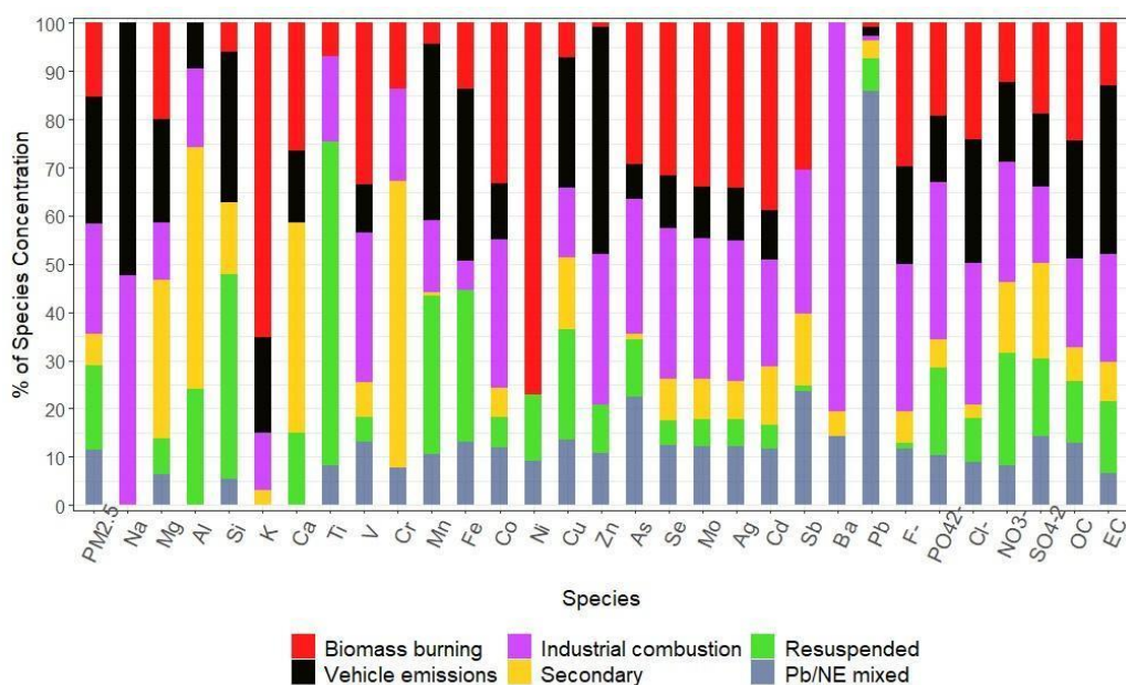
Figura 9. Perfil de fuentes en la estación de monitoreo el POLI Fuente: Preparado por los autores
