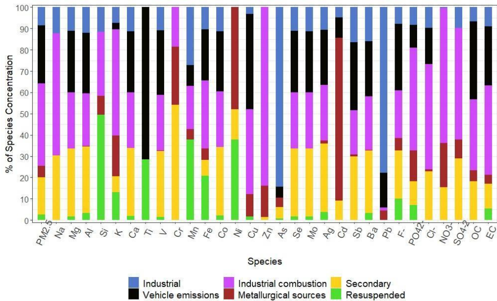
Figura 11. Huella de perfil de fuentes en la estación de monitoreo UPB. Fuente: Preparado por los autores
