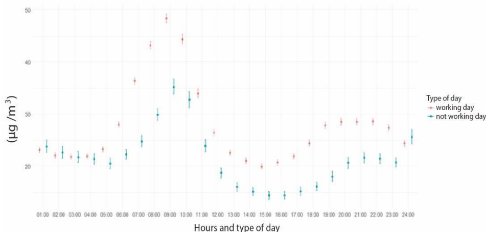
Figura 6. Intervalos de confianza PM_{2.5} por hora y tipo de día (Laboral y No Laboral) Valle de Aburrá, Colombia. 2009 - 2011. Fuente: Preparado por los autores.
