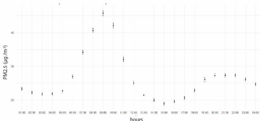
Figura 5. Comportamiento horario de PM_{2.5} ( \mu\text{g}/\text{m}^3 ). Valle de Aburrá, Colombia. 2009 – 2011. Fuente: Preparado por los autores.
