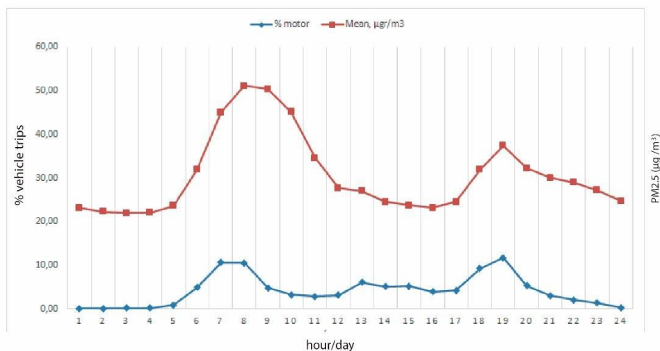
Figura 8. Distribución PM 2.5 (µg/m 3 ) promedio y viajes-hora/día. Valle de Aburrá, Colombia. 2009 – 2011.
