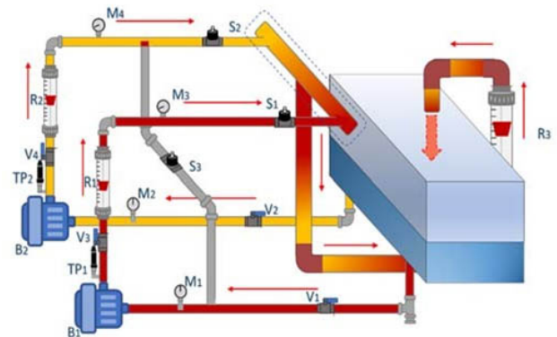
Fig. 4. Sistema de bombas centrífugas en paralelo.
