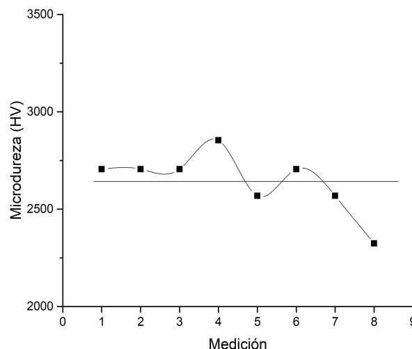
Fig. 6. Microdureza de la capa obtenida mediante TRD sobre la fundición nodular.
