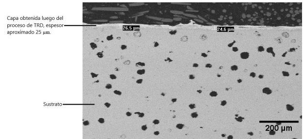
Fig. 3. Imagen de microscopía electrónica de barrido de la capa obtenida mediante difusión termorreactiva, sobre una fundición nodular (SEM, electrones retrodispersados (BSE)). La capa es homogénea en espesor.
