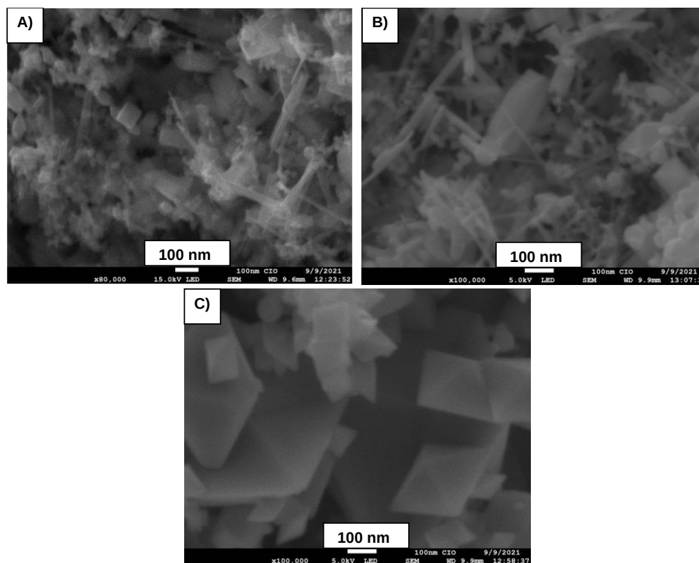
Fig. 6. Imágenes SEM de los polvos obtenidos por HFCVD en ambiente de: a) Ar, b) \text{Ar}+\text{H}_2\text{O} y c) Aire.
