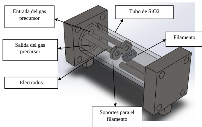
Fig. 1. Esquema del sistema de HFCVD.
