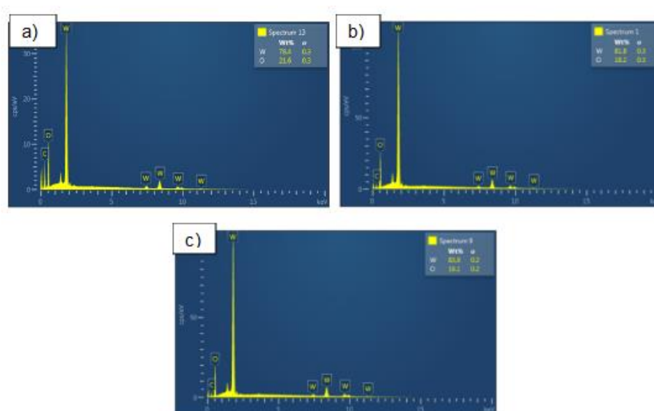
Fig. 7. Espectros EDS de los polvos de \text{WO}_3 obtenidos en ambiente de: a) Ar, b) \text{Ar}+\text{H}_2\text{O} y c) Aire.
