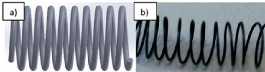
Fig. 3. a) Ilustración esquemática del filamento de tungsteno b) filamento utilizado para la deposición de \text{WO}_3 .
