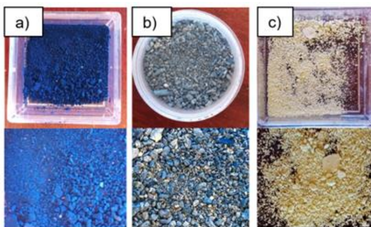
Fig. 4. Polvos obtenidos por la síntesis de HFCVD usando los gases: a) Ar, b) \text{Ar}+\text{H}_2\text{O} y c) Aire.
