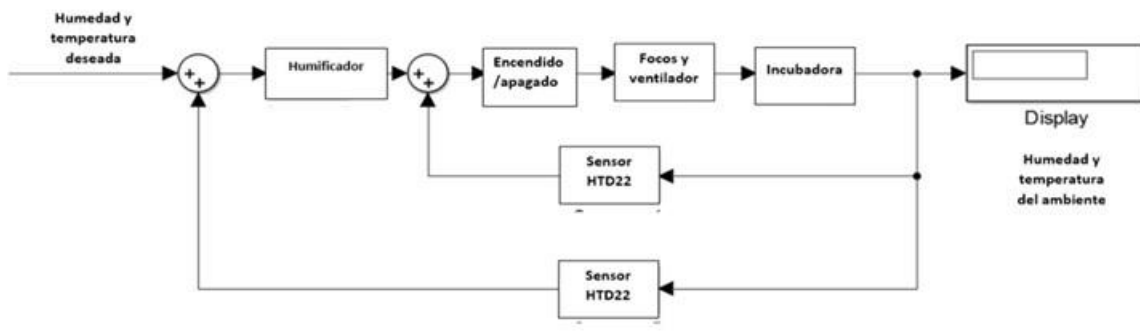
Fig. 4. Sistema de temperatura y humedad de lazo cerrado.
