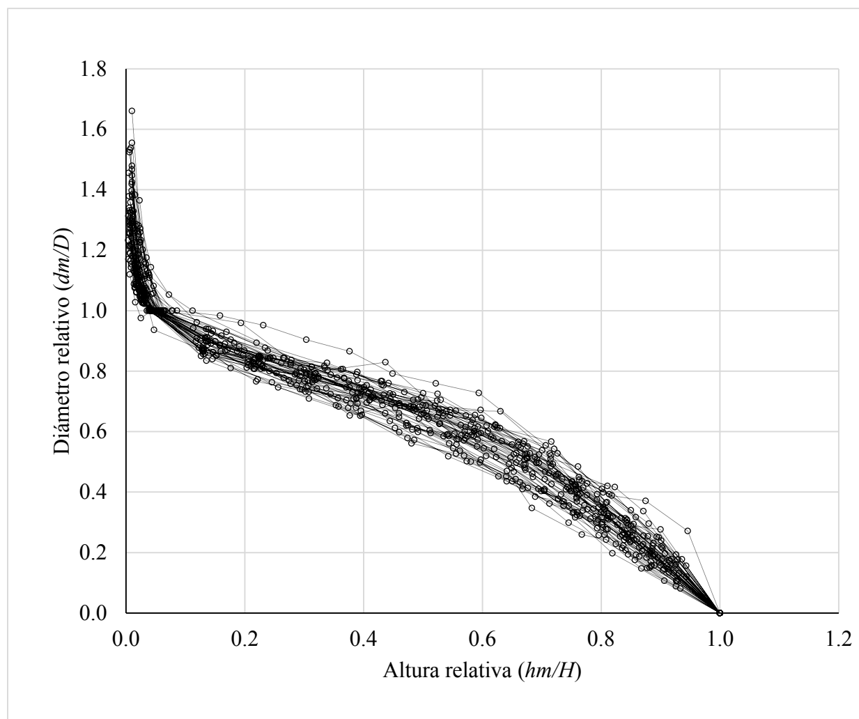
FIGURA 1. Dispersión del diámetro relativo y la altura relativa
