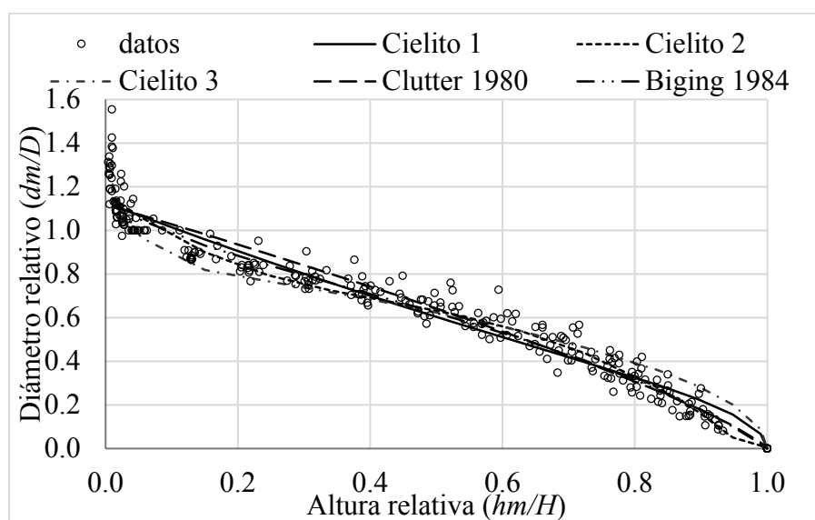
FIGURA 2. Comportamiento promedio de las cinco funciones de ahusamiento sobrepuestas a los datos de los perfiles fustales de P. ayacahuite .
