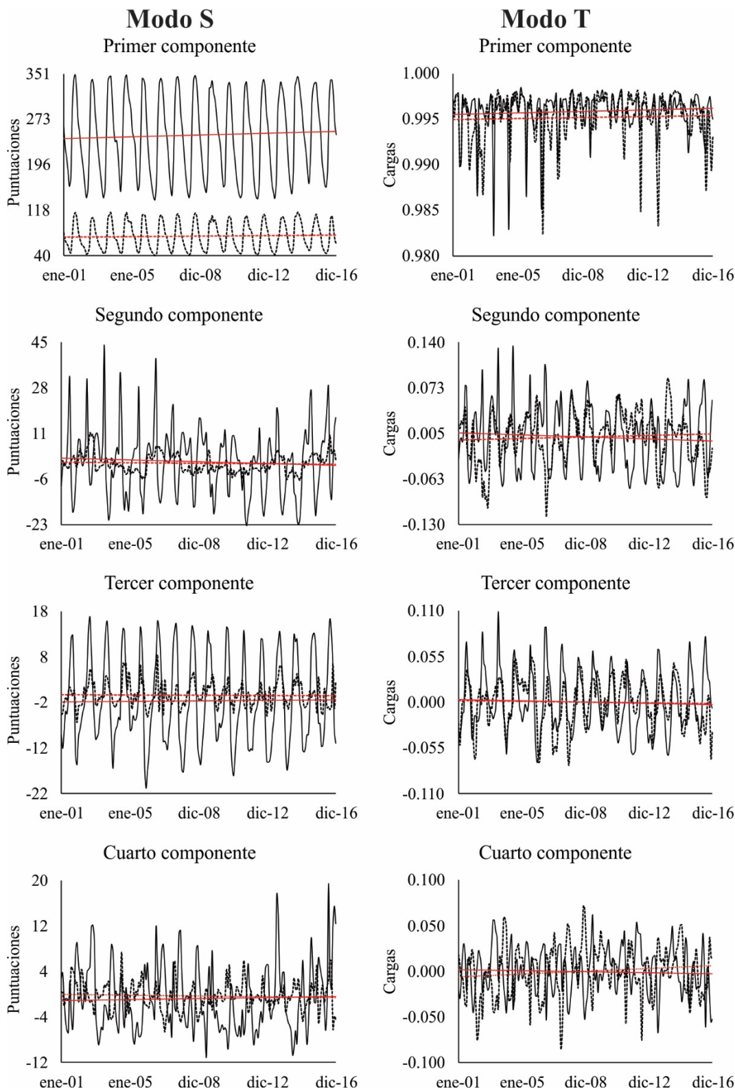
FIGURA 4. Perfiles de puntuaciones y cargas de los componentes del análisis de componentes principales con orientaciones en el modo S y T de una serie de tiempo mensual del NDVI de 2001 a 2016 en la cuenca Elota-Piaxtla-Quelite (línea sólida) y el Apffrmc (línea interrumpida).
