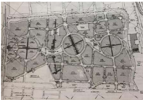
Figura 3. Ciudadela Colsubsidio. Planta general del proyecto
