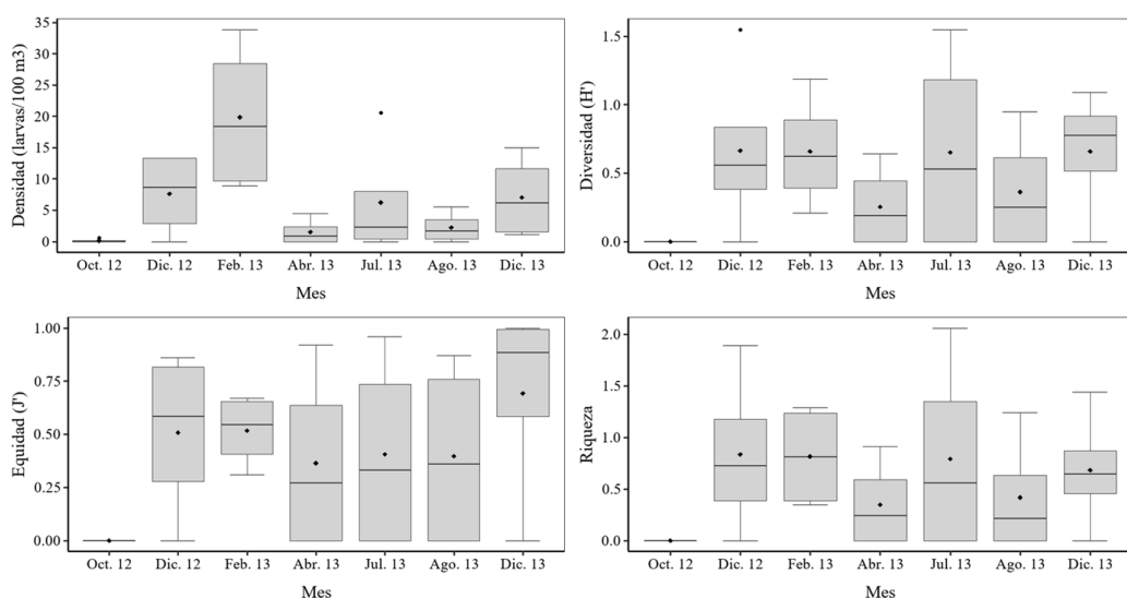
Fig. 4. Variación de la densidad de larvas (larvas/100 m 3 ) y los aspectos ecológicos diversidad (H'), equidad (J'), riqueza, en los meses de muestreo, en aguas superficiales de la fosa de Cariaco, estado Sucre, Venezuela
