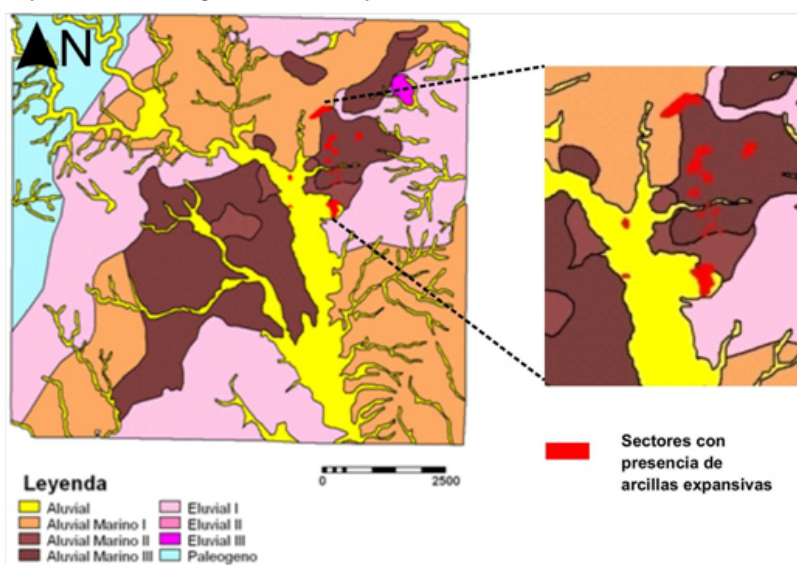
Figura 2. Mapa de pronóstico con la presencia de arcillas expansivas.
