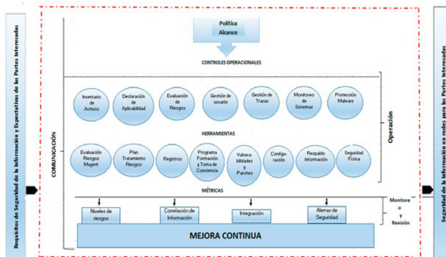
Figura 1. Modelo para la gestión de la seguridad de la información y los riesgos asociados a su uso en redes de computadoras
