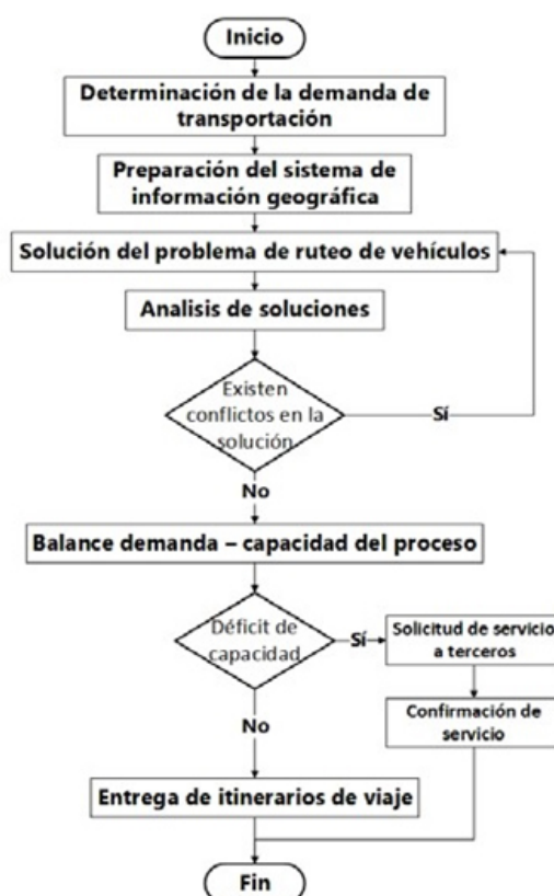
Figura 5. Procedimiento para la asignación de carga y planificación de rutas
