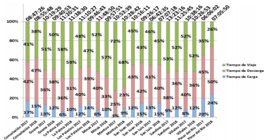
Figura 3. Estructura de los ciclos de transportación.
