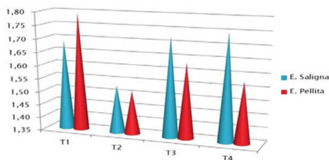
Figura 2. Valores medios de e Conicidad de las especies de Eucalyptus saligna Smith y en el Eucalyptus pellita F. Muell.
