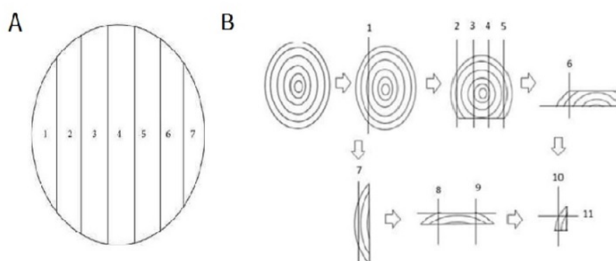
Figura 1. Métodos de aserrado.
