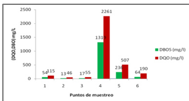
Figura 1. Comportamiento de la DBO 5 y la DQO en los diferentes puntos.
