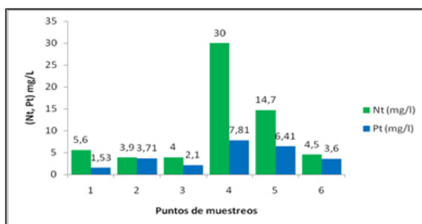
Figura 2. Comportamiento del nitrógeno total y fósforo total en los diferentes puntos.
