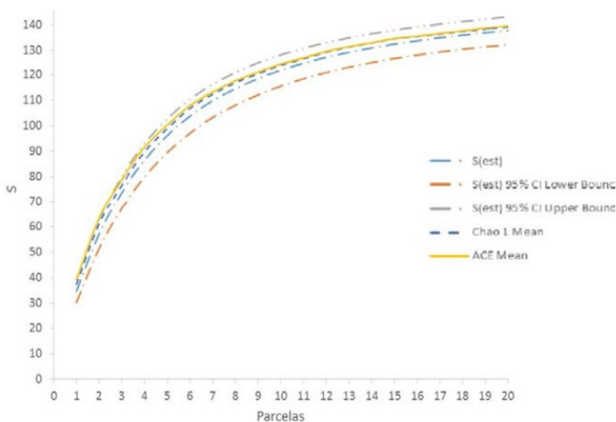
Figura 2. Curvas de acumulación de la riqueza observada.
