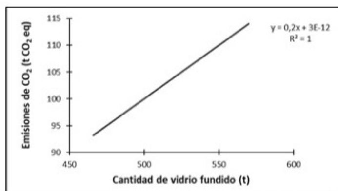
Figura 3. Emisiones de CO 2 y su relación con la cantidad de vidrio fundido.
