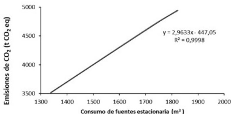
Figura 4. Emisiones de CO 2 y su relación con el consumo de fuentes estacionarias.
