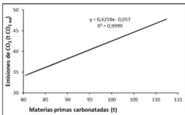
Figura 2. Emisiones de CO 2 y consumo de materias primas carbonatadas.
