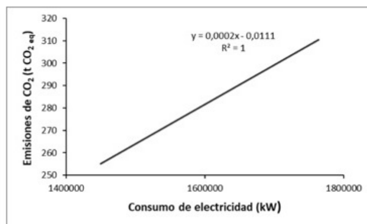
Figura 5. Emisiones de CO 2 y sus relación con el consumo de electricidad.
