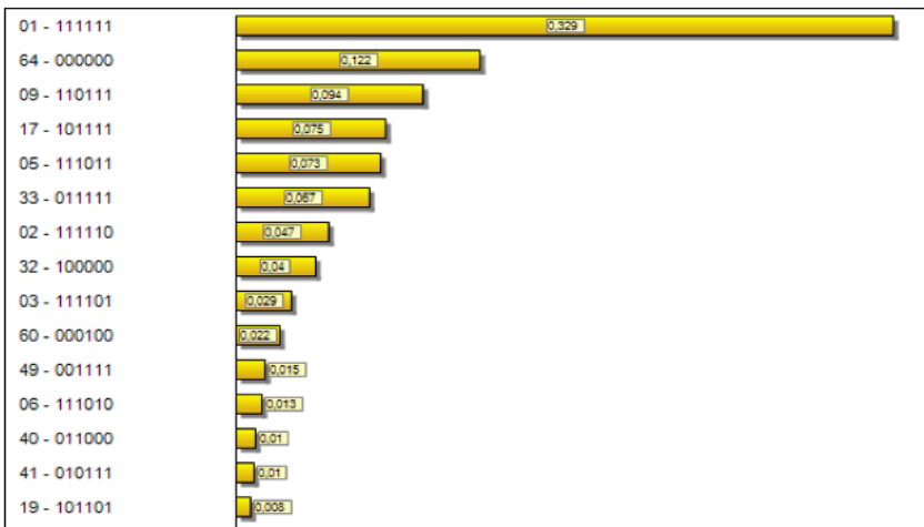
Figura 7. Histograma de probabilidades
