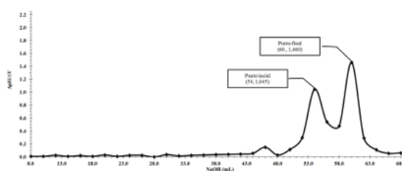
FIGURA 2 Grafica de la segunda derivada carboximetilquitosano (CMQ) frente a NaOH. de \Delta^2pH/\Delta V vs V (mL)
