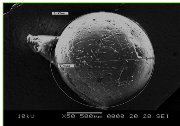
FIGURA 9. B Microfotografía de las esferas de hidrogel EDGE-PVA-Q con mediciones de circunferencia y dimensiones de la muestra
