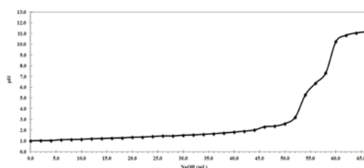
FIGURA 1 Curva de titulación del carboximetilquitosano (CMQ) frente a NaOH
