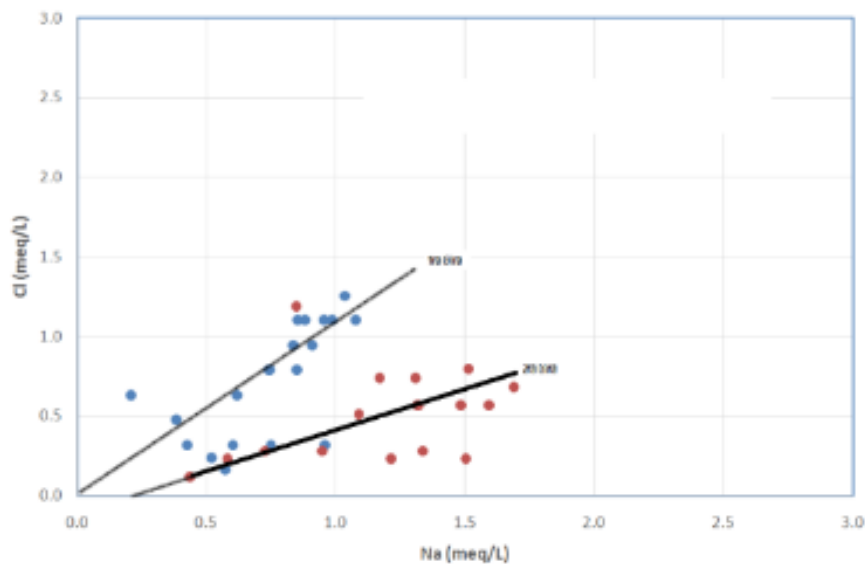
FIGURA 7 Relación de Na+ y Cl-. Ira y 2da Gira
