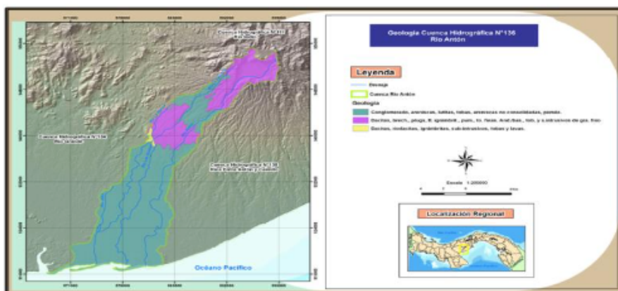
FIGURA 2 Geología de la Cuenca de Antón
