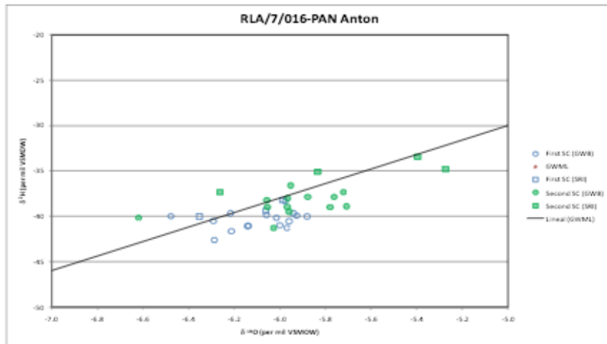
FIGURA 8 Recta Isotópica Antón 2013 y 2014
