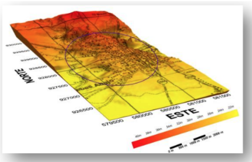
FIGURA 1 Mapa físico de la Ciudad de Antón
