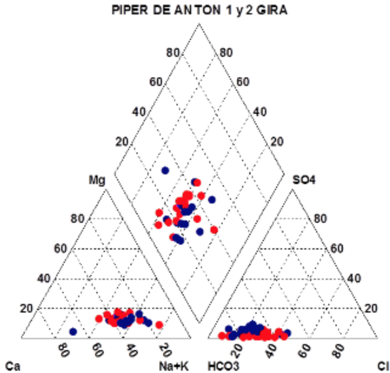
FIGURA 6 Diagrama Piper Gira 2013 y 2014
