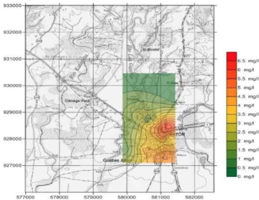
FIGURA 9 Nitratos (Gira 2013)
