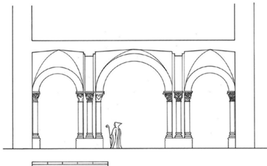
Fig. 10. Reconstrucción hipotética del acceso a la iglesia de Alfonso III en Sahagún desde el bloque occidental y panteón de Alfonso VI (J. L. Senra)
