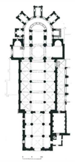
Fig. 11. Planta de la iglesia monástica de Saint-Philibert de Tournus (J. Henriet)
