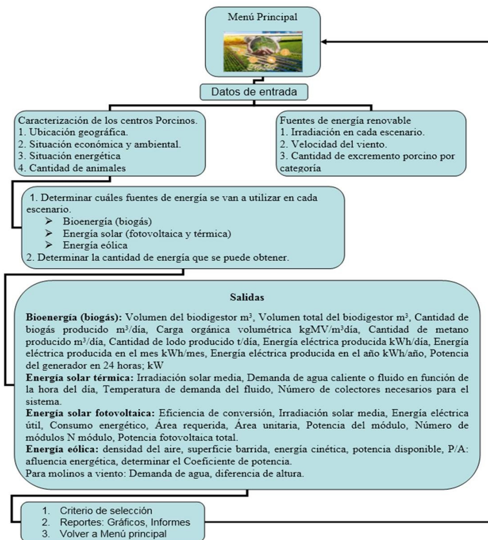
Figura 1. Esquema lógico-estructural del sistema informático FREAL
