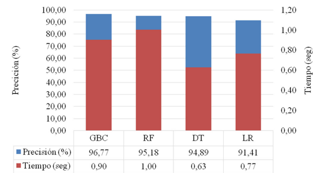
Figura 2. Precisión y tiempo de ejecución de los algoritmos de aprendizaje automático mejor valorados
