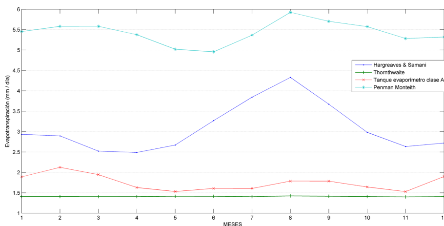
Figura 2. Distribución de valores obtenidos de ET_o para modelos de estimación (Thornthwaite, Hargreaves, Penman-Monteith y Tanque A).
