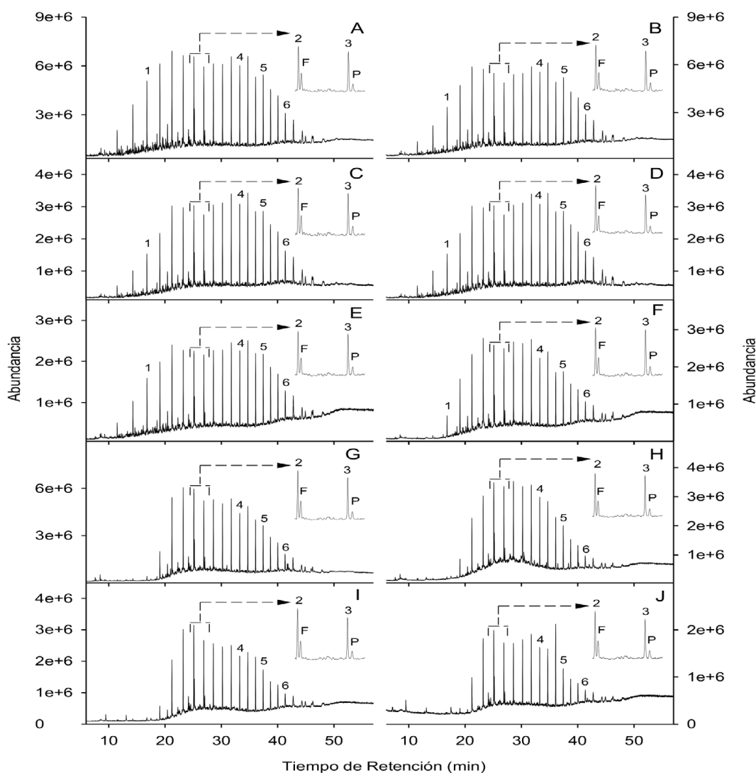
Figura 1. Cromatogramas de iones totales para los crudos extraídos de suelo a los tiempos T0 (A), T1 (B), T2 (C), T3 (D), T4 (E), T5 (F), T6 (G), T7 (H), T8 (I), T9 (J). 1: tridecano ( n\text{-C}_{13} ), 2: heptadecano ( n\text{-C}_{17} ), 3: octadecano ( n\text{-C}_{18} ), 4: docosano ( n\text{-C}_{22} ), 5: pentacosano ( n\text{-C}_{25} ), 6: octacosano ( n\text{-C}_{28} ), P: pristano, F: fitano.
