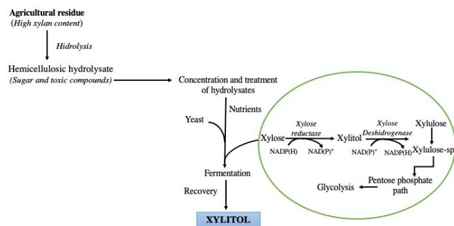
Figura 3. Producción biotecnológica de xilitol (Silva et al. 2004).
