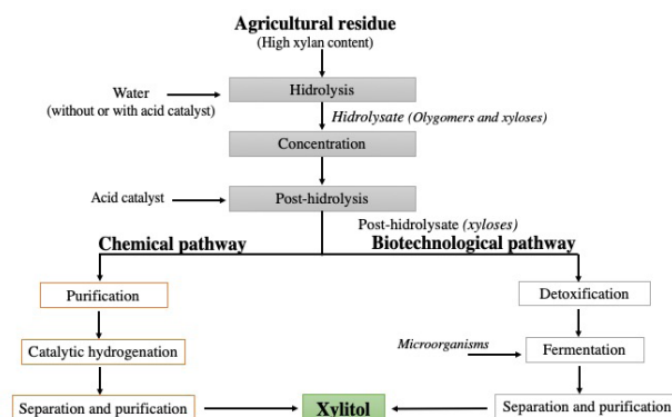
Figura 2. Producción de xilitol por ruta química y biotecnológica (Adaptado de Vallejos y Area, 2017).
