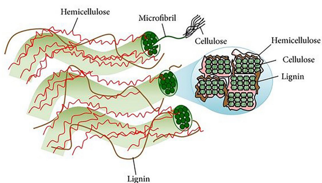
Figura 1. Estructura de la pared celular y sección transversal de las microfibrillas (cadenas de moléculas de celulosa incrustadas en un matriz de hemicelulosa y lignina). Adaptado de Lee et al. , 2014.
