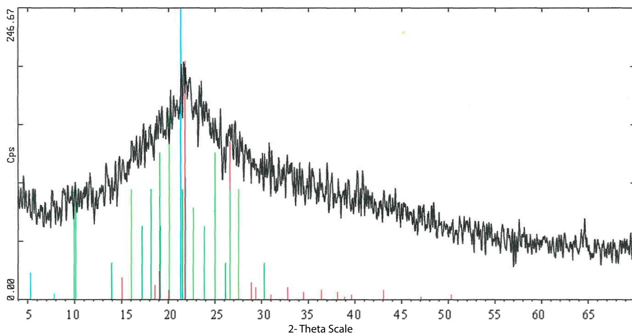
Figura 2. Difractograma de la composición química de las hojas de Mentha spicata L. nombre común hierbabuena. ■
