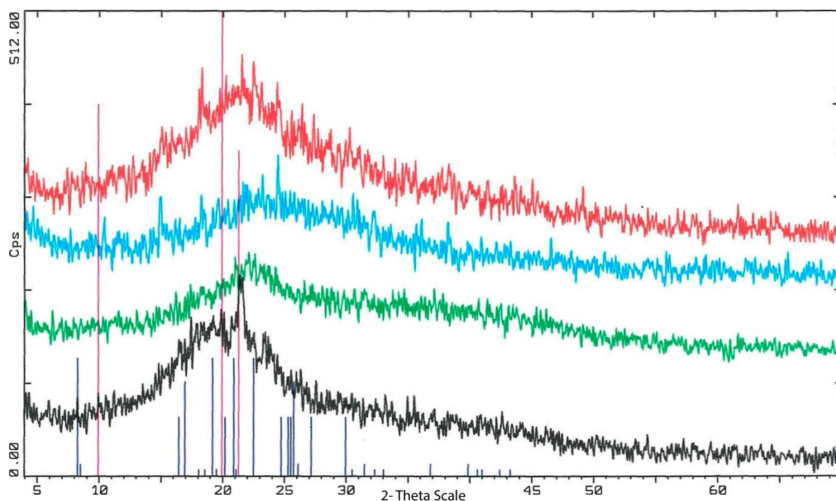
Figura 3. Difractograma de la composición química de las hojas de Ocimum basilicum L, nombre común Albahaca ■. Coriandrum
