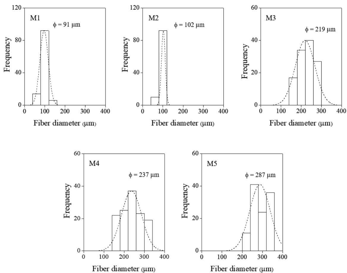
Figure 5. Normalized size distribution of raw PAN microfibers obtained with spinneret of inner diameters: a) 108 μm (M1), b) 127 μm (M2), c) 260 μm (M3), d) 311 μm (M4) y d) 337 μm (M5). Average fiber di-amer ( \phi ) is calculated from Gaussian fitting of the histograms. Figura 5. Distribución normalizada del tamaño de las microfibras crudas de PAN obtenidas con hilas de diámetros interiores: a) 108 μm (M1), b) 127 μm (M2), c) 260 μm (M3), d) 311 μm (M4) y d) 337 μm (M5). El diámetro medio de las fibras ( \phi ) se ha calculado a partir del ajuste gaussiano de los histogramas.
