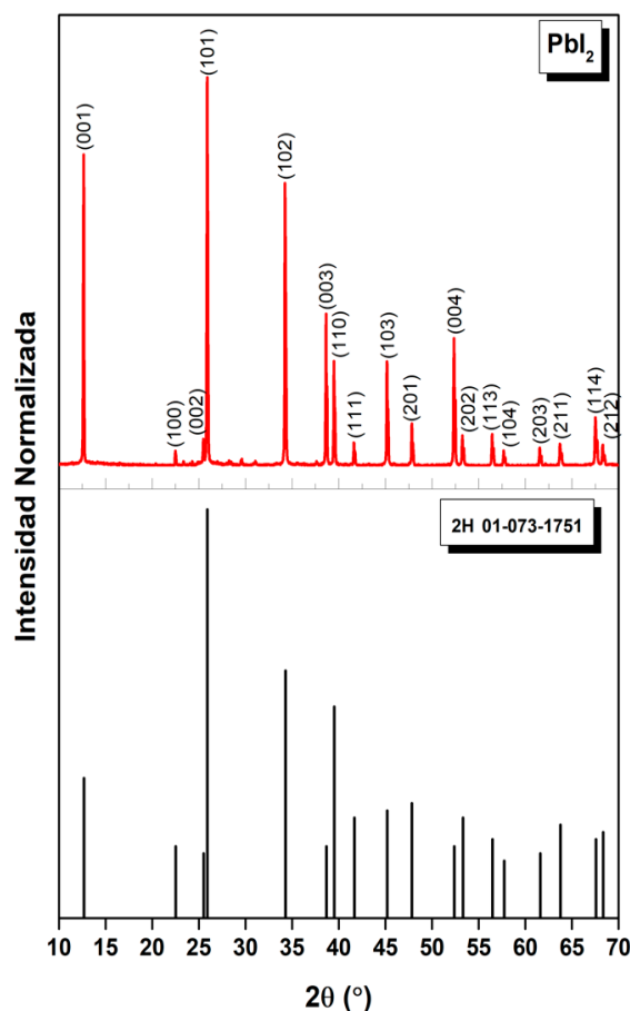
Figura 3. Patrón de difracción de rayos X de las nanopartículas de yoduro de plomo y carta cristalográfica JCPDS # 01-073-1751, correspondiente al politipo hexagonal de \text{PbI}_2 2H. Figure 3. X-ray diffraction pattern of lead iodide nanoparticles. JCPDS crystallographic card # 01-073-1751, corresponding to \text{PbI}_2 2H hexagonal polytype.
