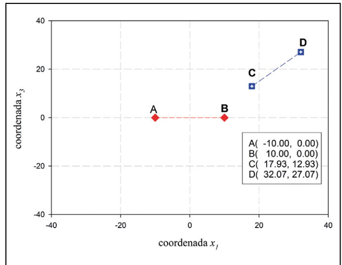
Figura 5. Orientación de receptores en un medio con una relación de Poisson \nu = 0.25 . Elaboración propia.
