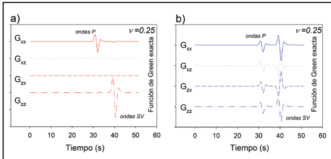
Figura 6. Funciones de Green exactas mediante sismogramas sintéticos. a) Receptores A y B; b) receptores C y D. Elaboración propia.
