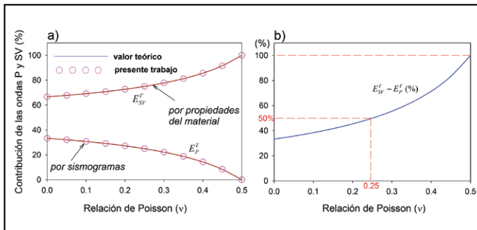
Figura 7. a) Contribución teórica de las ondas P y SV a la energía total; b) diferencia de E_{SV}^T - E_P^T en función de la relación de Poisson. Elaboración propia.
