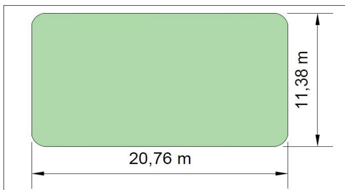
Figura 4. Laguna anaerobia con el método tradicional de diseño. Elaboración propia.
