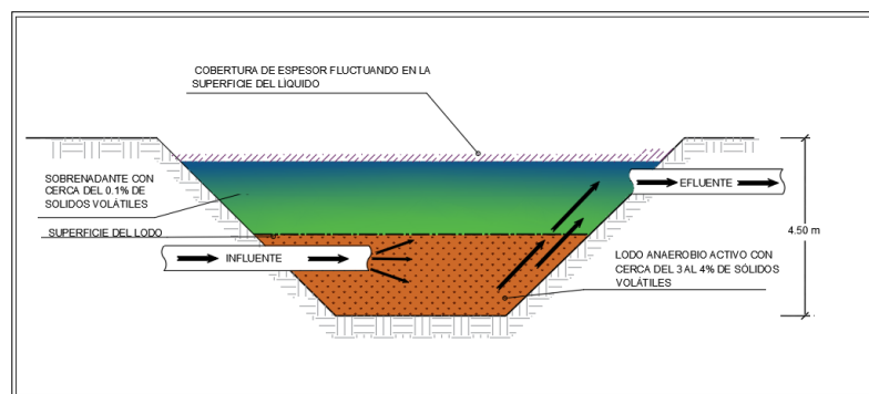
Figura 1. Tratamiento de una laguna anaerobia [Fotografía]. Imagen adaptada de Comisión Nacional del Agua & Instituto Mexicano de Tecnología del Agua (2016).
