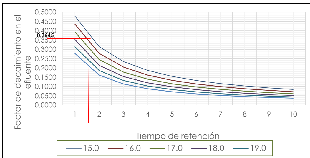
Figura 5. Ejemplo de aplicación del factor de cálculo para los coliformes fecales para temperaturas entre 15 y 20 °C en la eliminación de coliformes fecales. Elaboración propia.
