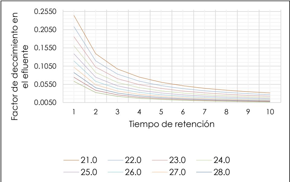
Figura 3. Curvas que corresponden a la ecuación (20) factor de cálculo para los coliformes fecales para temperaturas entre 21 y 30 °C. Elaboración propia.
