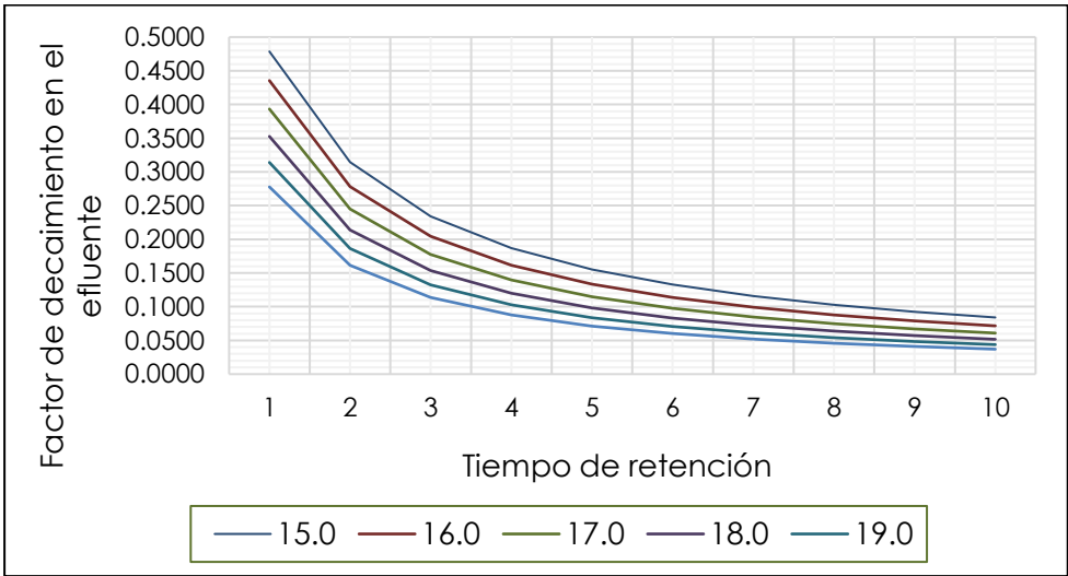
Figura 2. Curvas que corresponden a la ecuación (20) factor de cálculo para los coliformes fecales para temperaturas entre 15 y 20 °C en la eliminación de coliformes fecales. Elaboración propia.
