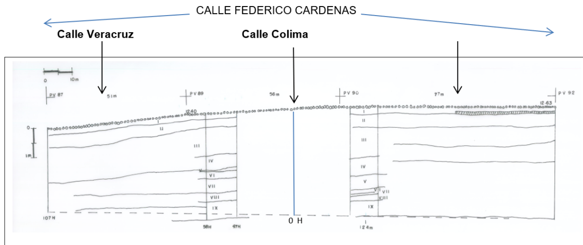
Figura. 3 Perfil estratigráfico donde se ubican las calles que cruzan la de Federico Cárdenas; la calle de Veracruz corresponde al número (107 - H); los números que van del cero (0) a la letra (H) inician en el centro de la calle de Colima hacia la calle de Veracruz, que corresponde al número (107 - H). Fuente: Jiménez (2017).
