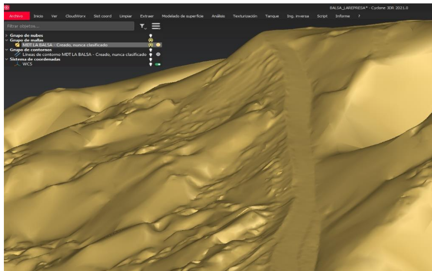
Ilustración 5. Modelo digital de terreno, nube de puntos procesada, sin las copas de los arboles
