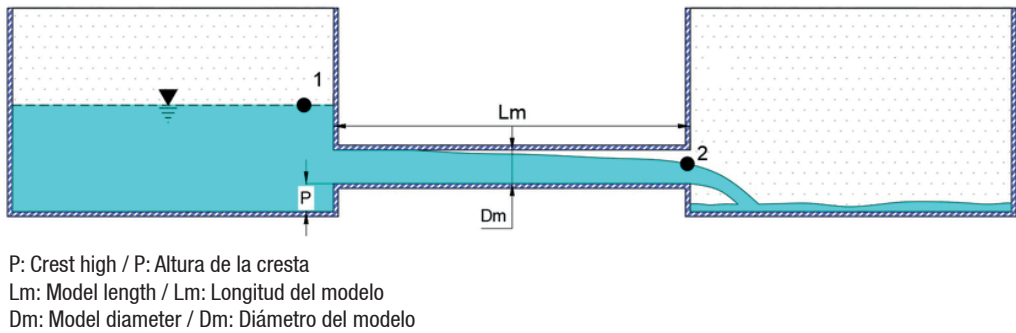
Figure 1. Conceptual scheme of the culvert-type physical model. Figura 1. Esquema conceptual del modelo físico tipo alcantarilla.
