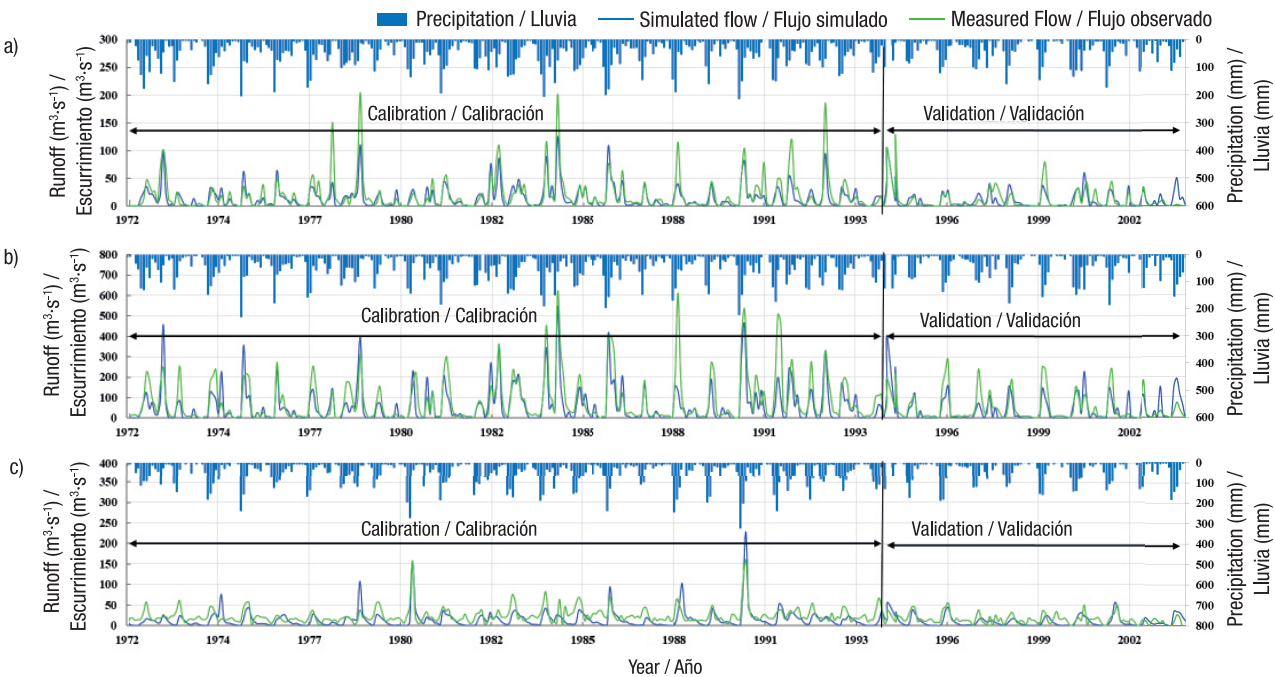
Figure 4. Measured vs simulated runoff by SWAT for the calibration and validation of three sub-watersheds: a) Angostura, b) El Novillo and c) El Oviachic. Figura 4. Escorrimento observado vs simulado por SWAT para la calibración y validación de tres subcuencas: a) Angostura, b) El Novillo y c) El Oviachic.
