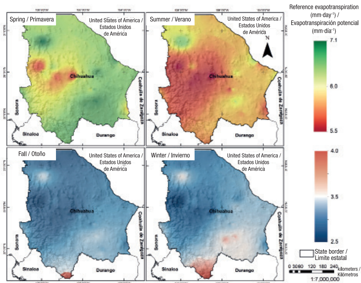
Figure 9. Spatial distribution of reference evapotranspiration ( ET_0 ) estimated by the Hargreaves method (1960-2013). Figura 9. Distribución espacial de evapotranspiración de referencia ( ET_0 ) por el método Hargreaves (periodo 1960-2013).
