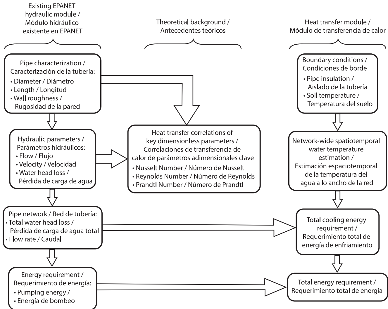
Figure 1. Flowchart to develop a heat transfer module in conjunction with existing EPANET hydraulic module. Figura 1. Diagrama de flujo para desarrollar un módulo de transferencia de calor junto con el módulo hidráulico existente en EPANET.
