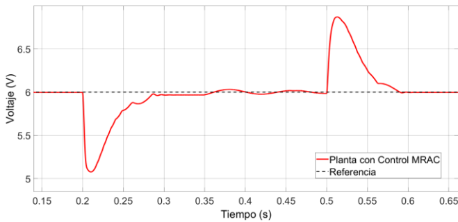
Figura 5. Respuesta en estado estacionario a cambios del voltaje de alimentación
