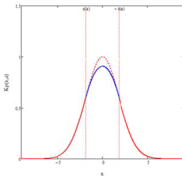
2 pav Keplerio parabolė (mėlyna spalva).
