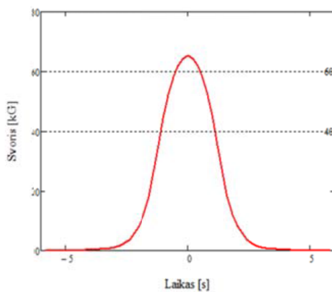
3 pav 70 kg masės MT svoris judant parabole.
